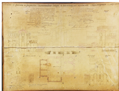
4. სამთავისის ეკლესიის პროექტი. არქიტექტორი ფრანსუა ქსავიე რიპარდი. საქართველოს ეროვნული არქივი, საისტორიო ცენტრალური არქივი. ფონდი 205, საქმე 2125 (1847 წელი).
